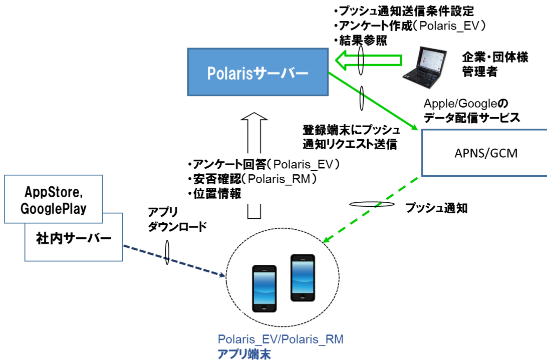
図1 システム構成 (Polaris_EV)
