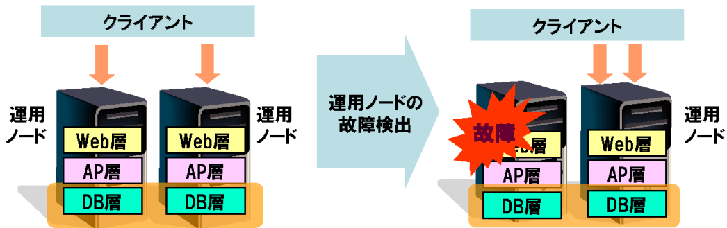
「DBC/APKeeper+DB/Control」による両系運用のノード構成
